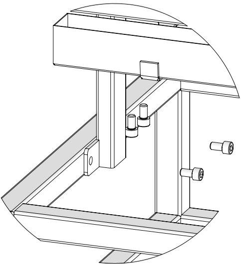
DETAIL AY SCALE 1 : 4
